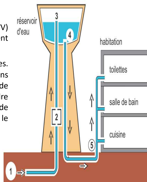
Schéma d'un château d'eau
